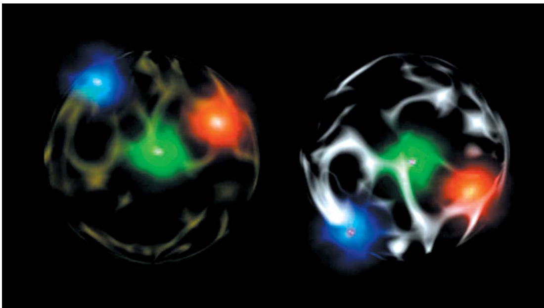
Gell-Mann đề xuất rằng các hạt như proton, neutron được tạo nên từ các quark. Ảnh: Cassiopeia Project.
